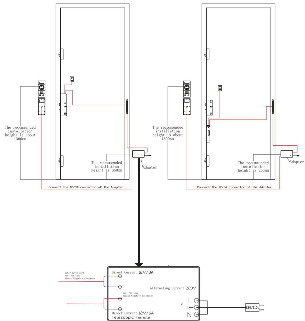
Увеличенная схема блока питания
