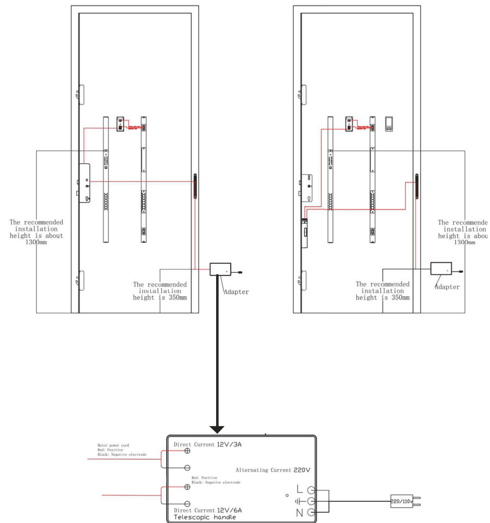
Увеличенная схема блока питания
